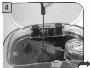
Открутите винт, удерживающий сервисную дверцу в закрытом состоянии.
